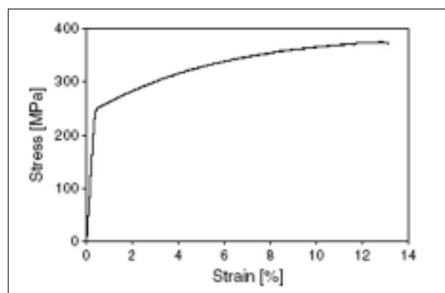
FIG. 4 Curva tensione-deformazione ingegneristica.
