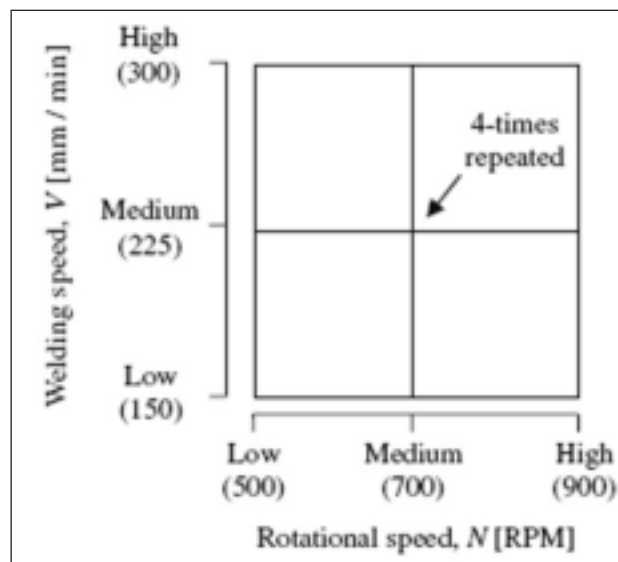
FIG. 2 Piano fattoriale 3 2 utilizzato nella campagna sperimentale.
