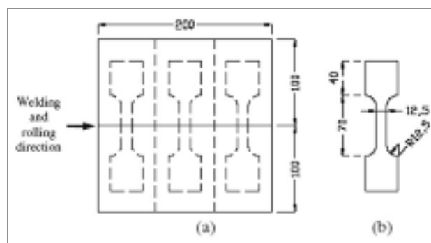
FIG. 1 (a) posizione dei provini rispetto alla direzione di saldatura e laminazione; (b) dimensione dei provini secondo ASTM E8M-04 (tutte le dimensioni sono in 'mm').
